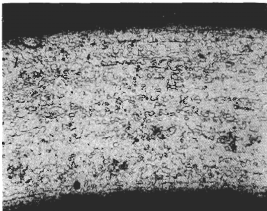
X 100 mag. Ferrite and slag
